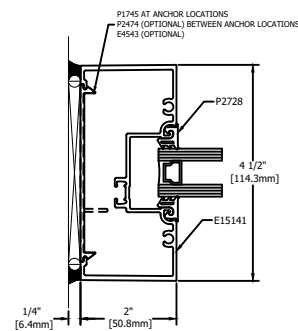
7 JAMB STANDARD
