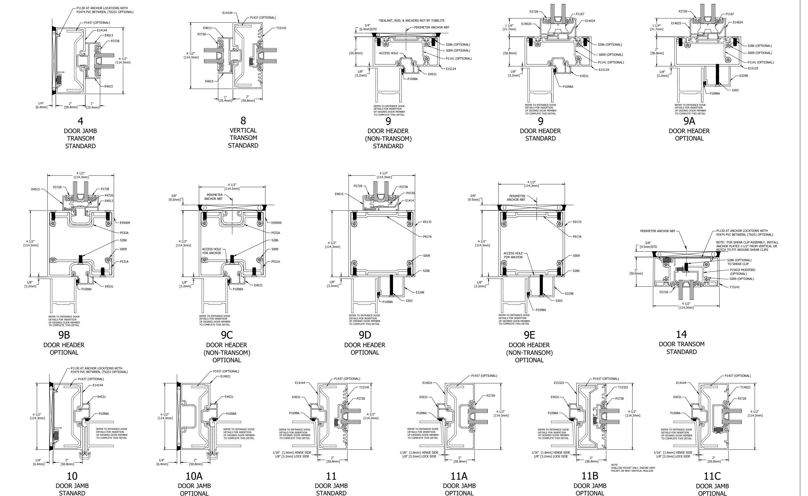
DOOR DETAILS
