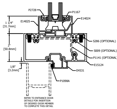
9 DOOR HEADER STANDARD
