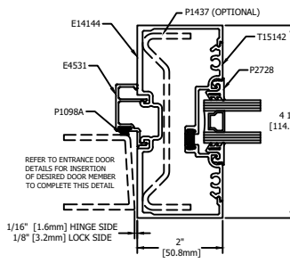
11 DOOR JAMB STANDARD
