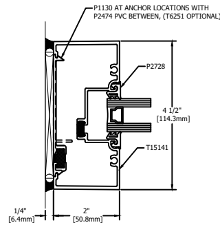
7 JAMB STANDARD
