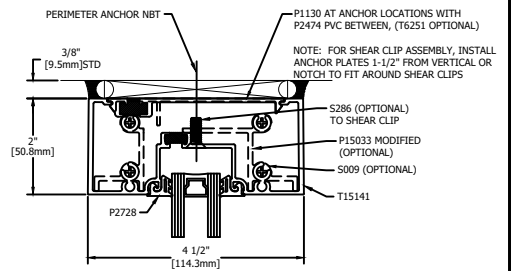
14 DOOR TRANSOM STANDARD
