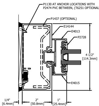
4 DOOR JAMB TRANSOM STANDARD
