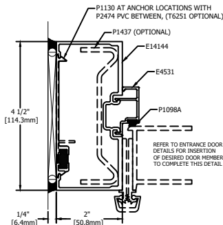
10 DOOR JAMB STANDARD
